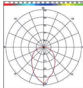
OTTICA 90°
