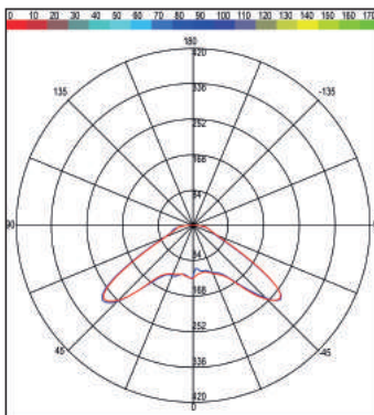
OTTICA 130°
