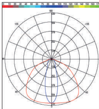
OTTICA 30°x 120°
