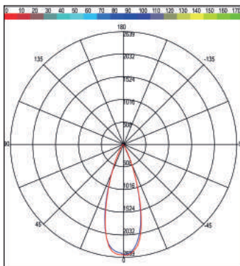
OTTICA 34°
