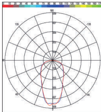
OTTICA 60°
